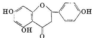
Kaempferol
